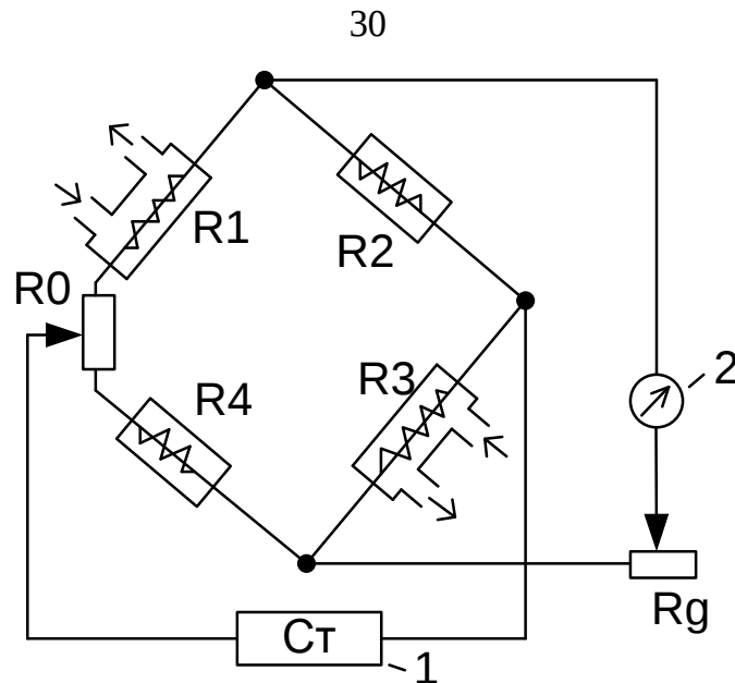
1 – источник стабилизированного напряжения; 2 – вторичный прибор; R_1 и R_3 – рабочие терморезисторы; R_2 и R_4 – сравнительные терморезисторы; R_0 и R_g – потенциометры; вход и выход анализируемой газовой смеси показаны стрелками.
