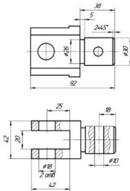
5 вариант. Деталь трубопровода.
