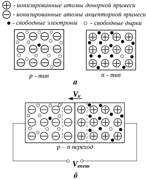
Рис. 2. Модель образования p-n перехода:
