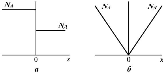
Рис. 1. Распределение концентрации акцепторов N_A и доноров N_D в р-п переходе: а – резком (ступенчатом); б – плавном
