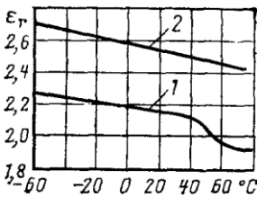
Рис. 7. Зависимость \epsilon от температуры для непольных диэлектриков; 1 – парафин; 2 – полистирол
