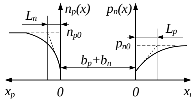
Рис. 8. Распределение концентрации неосновных носителей заряда в нейтральных областях вблизи р-п перехода при обратном включении: n_{p0} и p_{n0} – равновесные концентрации электронов и дырок в р- и n-областях; L_n и L_p – их диффузионная длина соответственно
