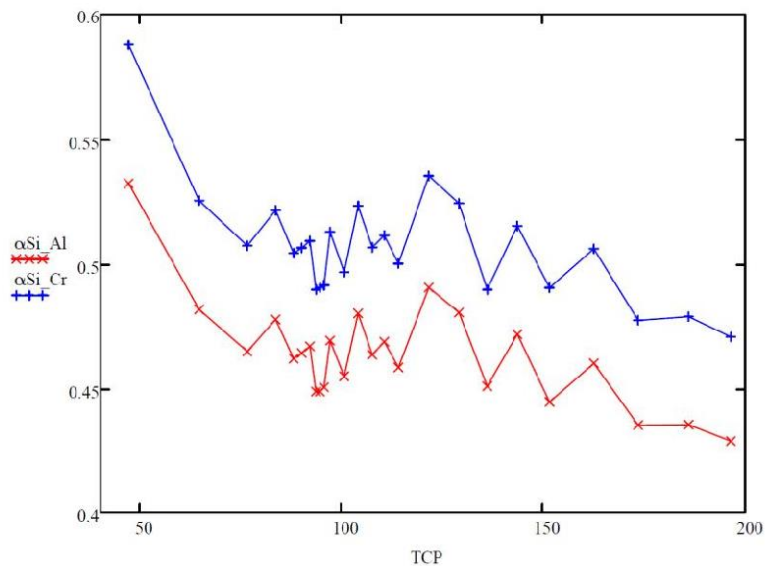
Температурная зависимость коэффициента термо-ЭДС, мВ/град
