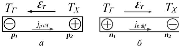
Рис. 1. Возникновение термо-ЭДС в полупроводниках: a – полупроводник n-типа; б – полупроводник p-типа ( T_\Gamma > T_X , p_1 > p_2 , n_1 > n_2 )
