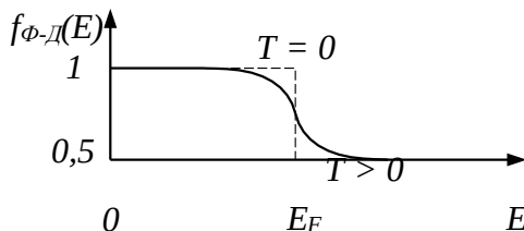
Рис. 6. Функция распределение Ферми – Дирака для электронов
