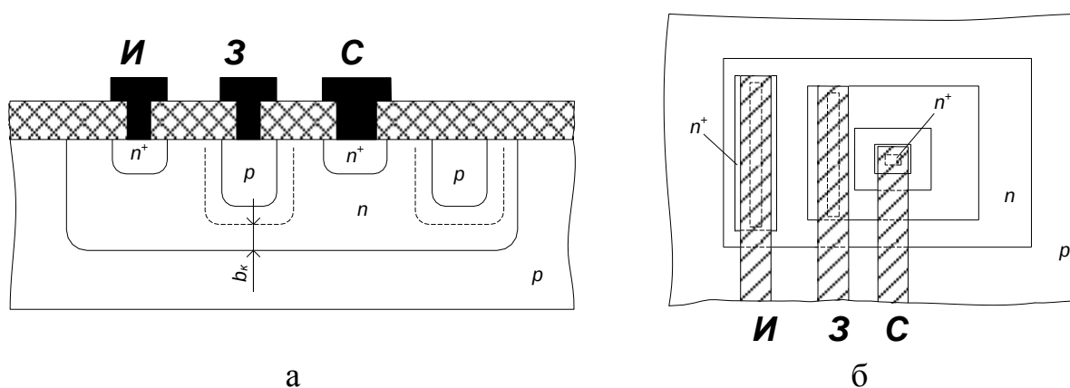
Рис. 1.8. Конструкция (а) и топология (б) полевого транзистора
