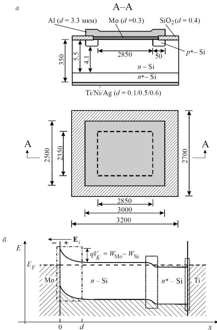
Рис. 4. Диод Шоттки: a – виды в плане и разрезе (размеры даны в мкм, S \approx 6.7 \text{ мм}^2 ); b – энергетическая зонная диаграмма
