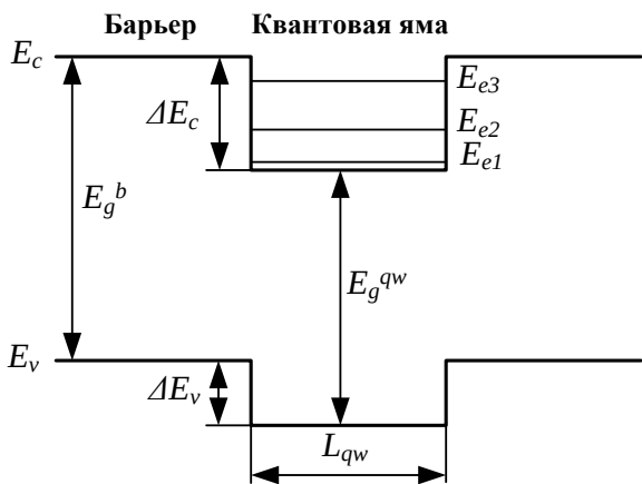
Рис. 3. Энергетическая диаграмма КРС с КЯ и зонной диаграммой I типа (а) и II типа (б)
