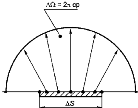
Рис. 3. Определение светимости [1]
