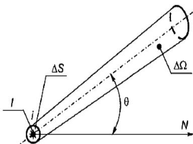
Рис. 4. Определение яркости [1]
