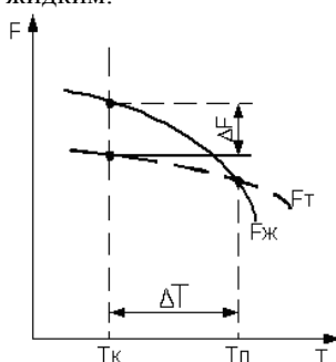
Рис. 1.9. Изменение энергии Гельмгольца F (свободной энергии) металла в жидком F_{ж} и твердом F_{т} состояниях в зависимости от температуры ( T_k — температура, при которой происходит кристаллизация)
