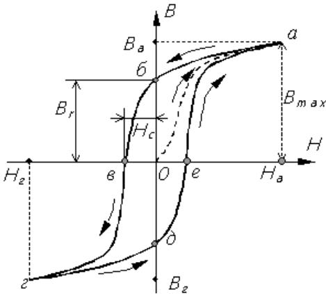
Рис. 1. График перемagnetизации ферромагнетиков (петля гистерезиса)
