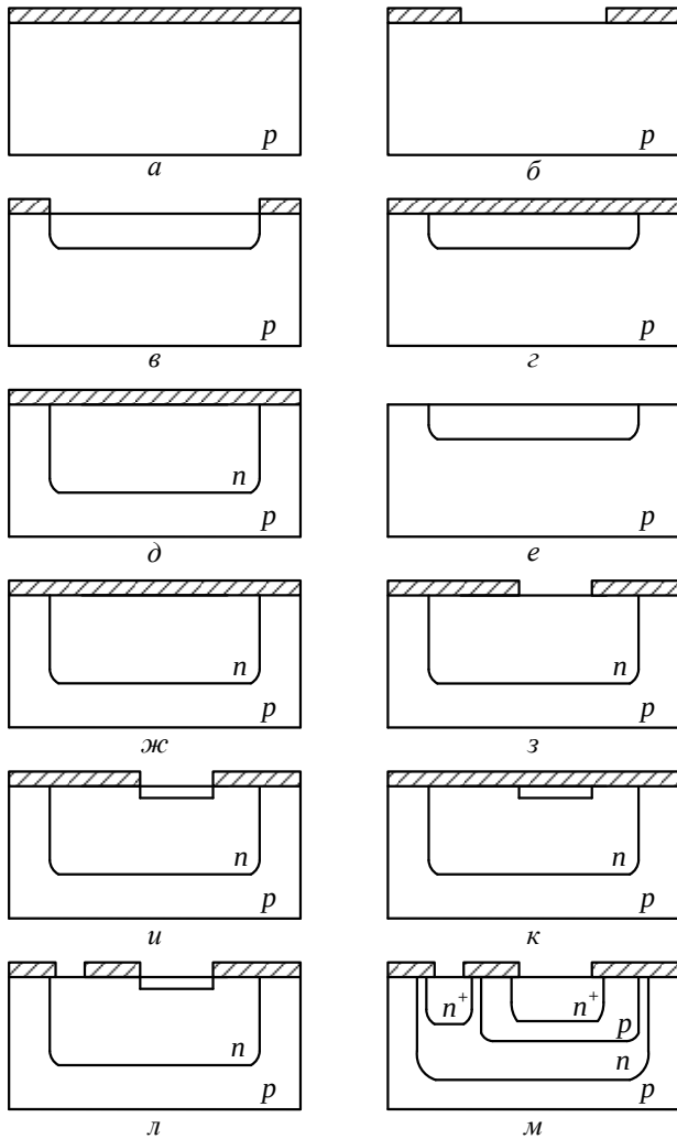
Рис. 3.1. Основные технологические этапы формирования интегрального биполярного транзистора n - p - n -типа: a – окисление, б – фотолитография коллекторного слоя, в – загонка коллекторной примеси, г – окисление, д – разгонка коллекторной примеси, е – травление, ж – окисление, з – фотолитография базового слоя, и – загонка базовой примеси, к – окисление, л – фотолитография эмиттерного слоя, м – загонка эмиттерной примеси и разгонка базовой примеси
