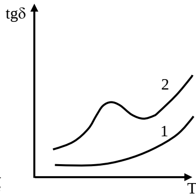
Рис. 5. Зависимость \text{tg}\delta от температуры для непольярных (1) и полярных (2) диэлектриков
