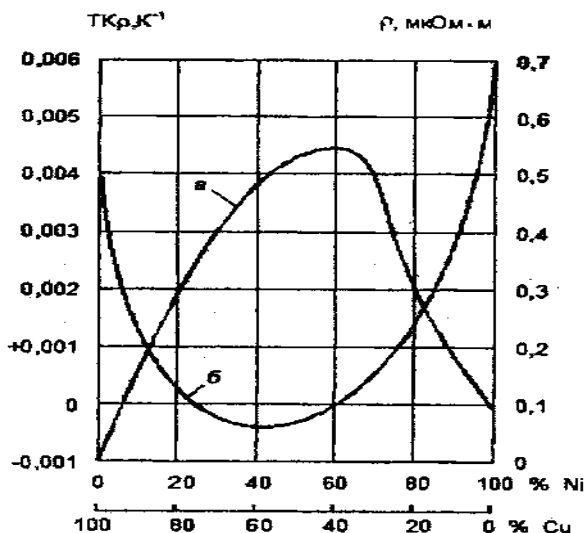
Рис. 4. Зависимость \rho (а) и TKR (б) сплавов системы Cu-Ni от состава (в процентах по массе) [1]
