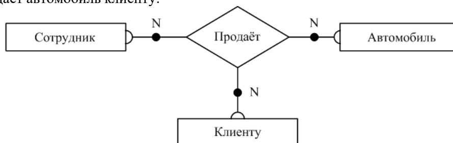
Рисунок 4 – ER-диаграмма связи «Сотрудник продаёт автомобиль клиенту»
