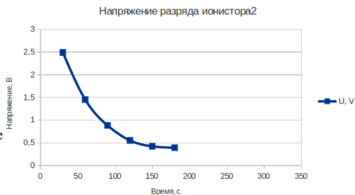
График напряжения разряда ионистора после прерывания процесса его разряда.
