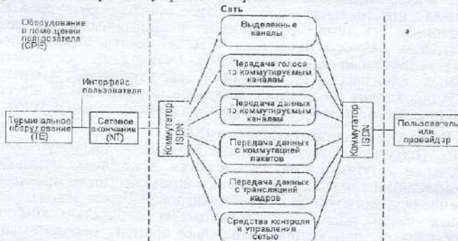
Рис. 1.1. Службы ISDN
