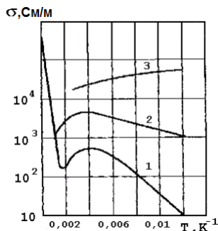
Рис. 2. Температурная зависимость удельной электрической проводимости кремния, содержащего различное количество донорной примеси N_D :
