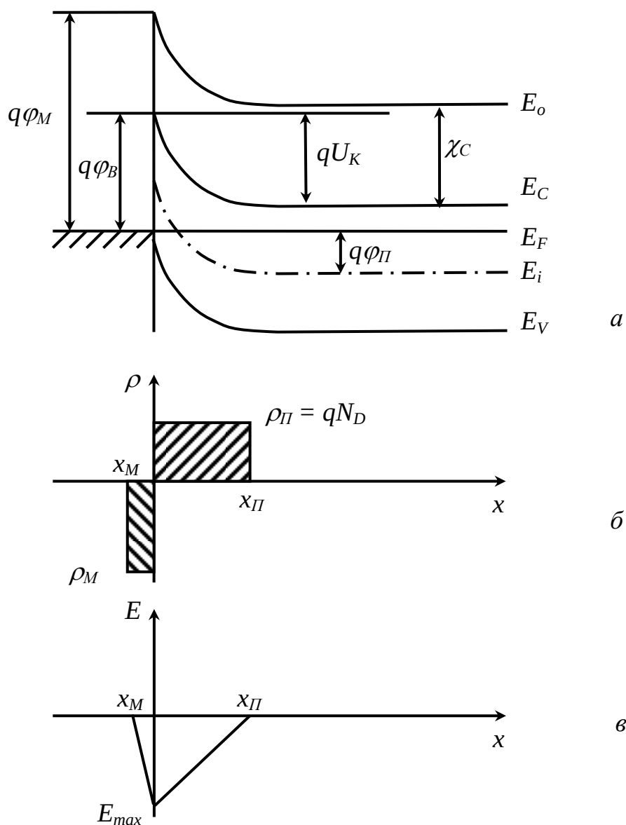
Рис. 2. Энергетическая зонная диаграмма контакта металл-полупроводник в равновесии (а); распределение заряда (б) и электрического поля (в); x_M и x_\Pi – границы СОЗ в металле и полупроводнике соответственно
