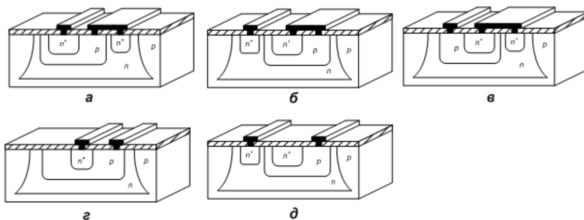
Рис. 1.7. Конструкции интегральных диодов: а – на основе перехода база-эмиттер с коллектором, закороченным на базу (БК-Э); б – на основе перехода коллектор-база с эмиттером, закороченным на базу (БЭ-К); в – с использованием эмиттерного и коллекторного переходов, когда эмиттерные и коллекторные области соединены (Б-ЭК); г – на основе перехода база-эмиттер с разомкнутой цепью коллектора (Б-Э), д – на основе перехода база-коллектор с разомкнутой цепью эмиттера (Б-К)
