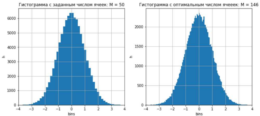
Рис. 9.5. Гистограммы
