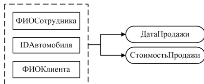
Рисунок 15 – Отношение «Продажа»
