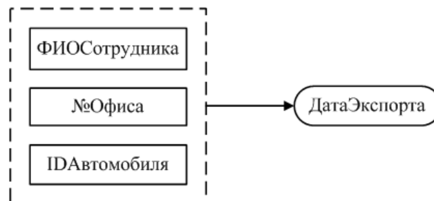
Рисунок 14 – Отношение «Экспорт»
