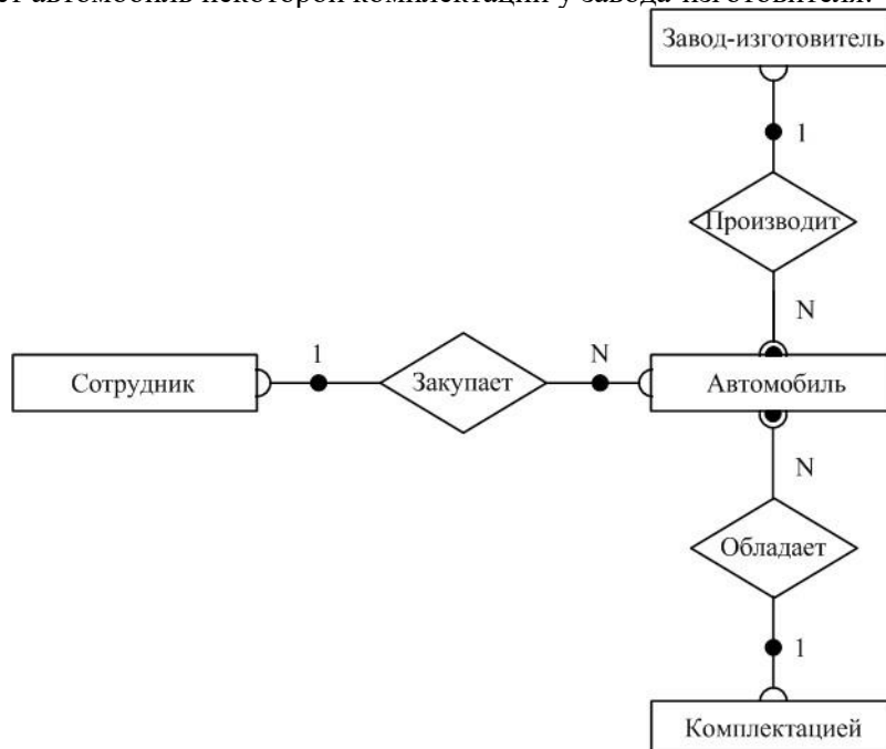
Рисунок 2 – ER-диаграмма связи
