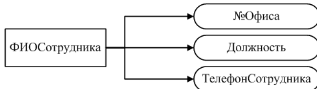
Рисунок 8 – Отношение «Сотрудник»
