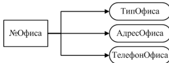
Рисунок 7 – Отношение «Офис»
