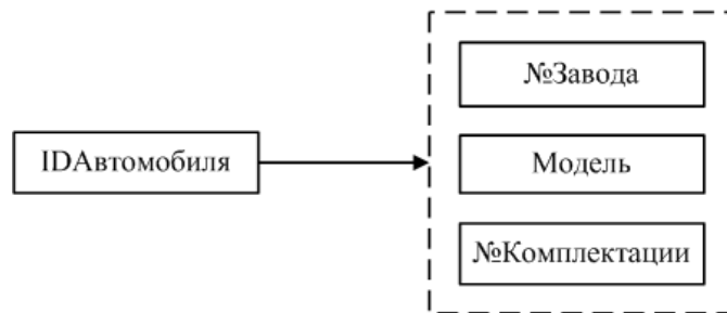
Рисунок 11 – Отношение «Автомобиль»
