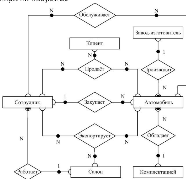
Рисунок 6 – Общая ER-диаграмма
