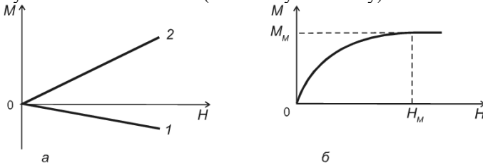
Рис. 2. Зависимость намагниченности M от напряженности магнитного поля H : а - для диамагнетиков (1) и парамагнетиков (2); б - для парамагнетиков при низких температурах или очень сильных полях
