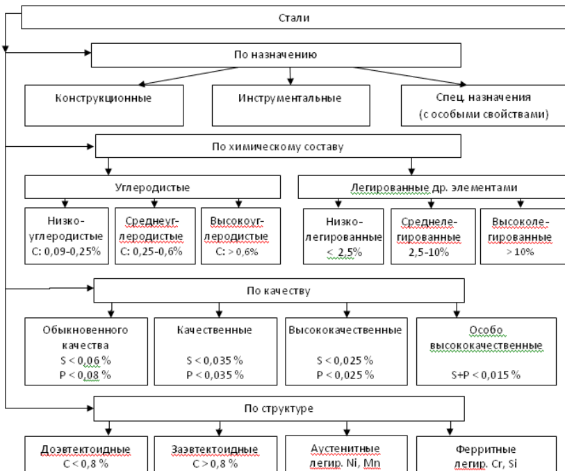
Рис. 2.4. Классификация сталей
