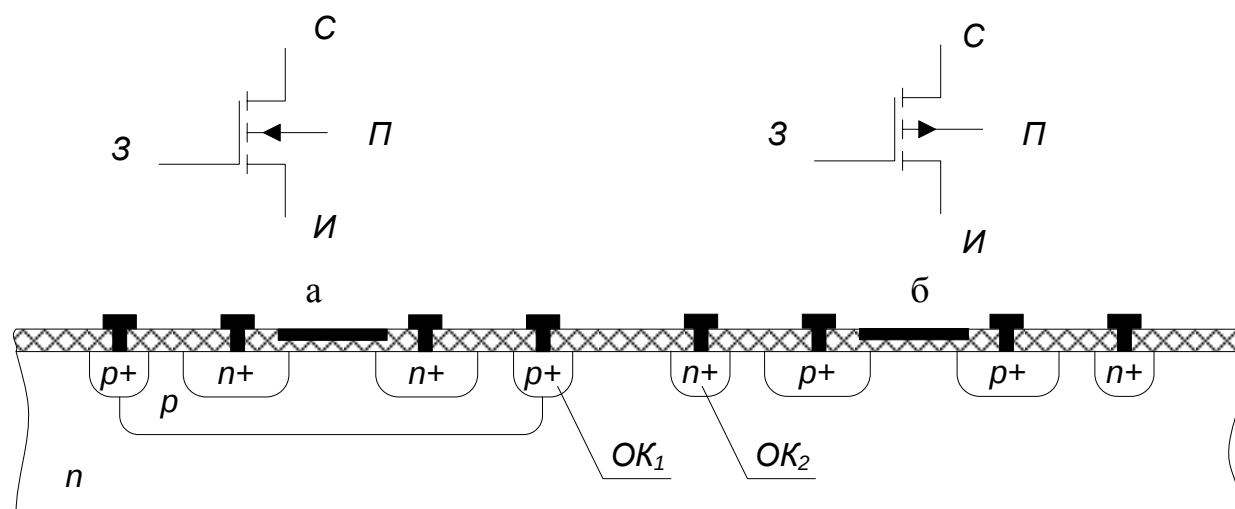
В Рис. 1.10. Конструкция МДП-транзисторов: а – п-МДП-транзистор; б – р-МДП-транзистор; в – комплиментарная пара транзисторов: ОК 1 , ОК 2 – охран- ные кольца
