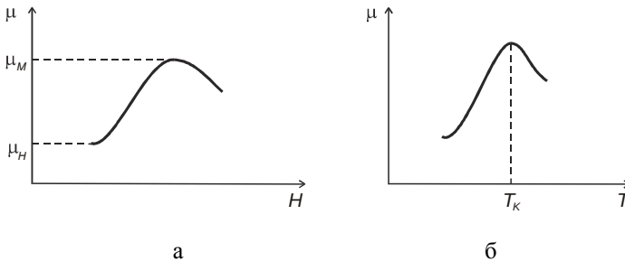
Рис. 2.4. Зависимость относительной магнитной проницаемости ферромагнетиков от напряженности магнитного поля (а) и температуры (б)
