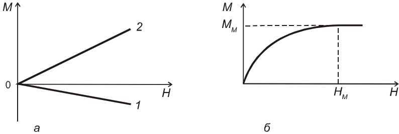
Рис. 1.4. Зависимость намагниченности M от напряженности магнитного поля H : a – для диамагнетиков (1) и парамагнетиков (2); б – для парамагнетиков при низких температурах или очень сильных полях
