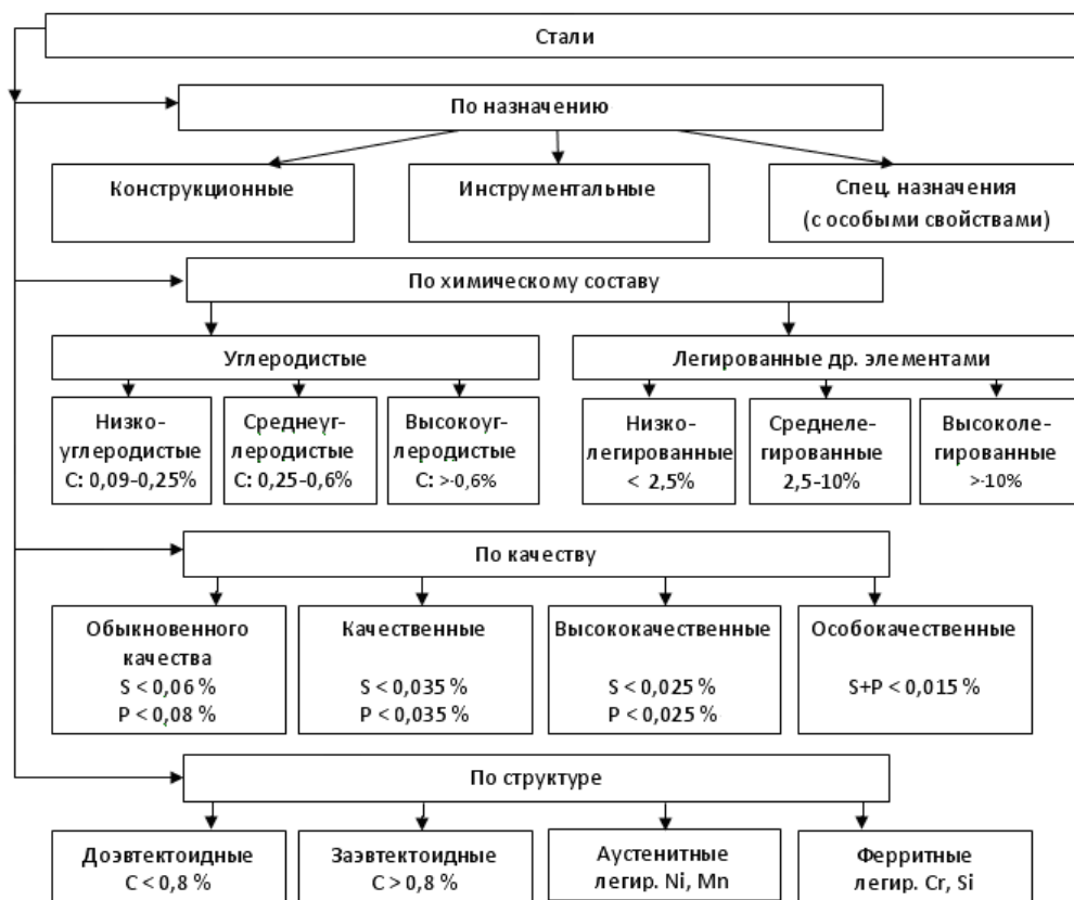
Рис. 1.5. Классификация сталей
