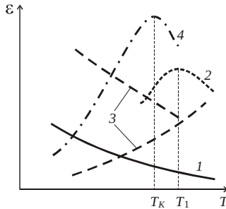
Рис. 1.7. Зависимость \varepsilon от температуры для диэлектриков с электронной (1), дипольно-релаксационной (2), ионной и ионно-релаксационной (3) и спонтанной (4) поляризацией
