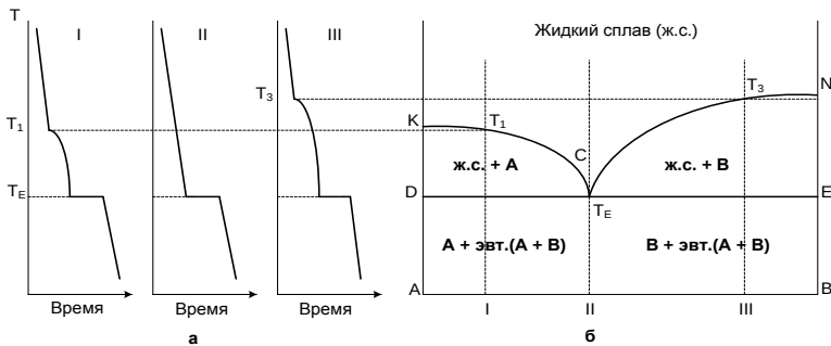
Рис. 1.2. Кривые охлаждения с концентрацией компонентов I, II, III (а) и диаграмма состояния сплавов, образующих в твердом состоянии сплав типа механической смеси компонентов A и B (б)
