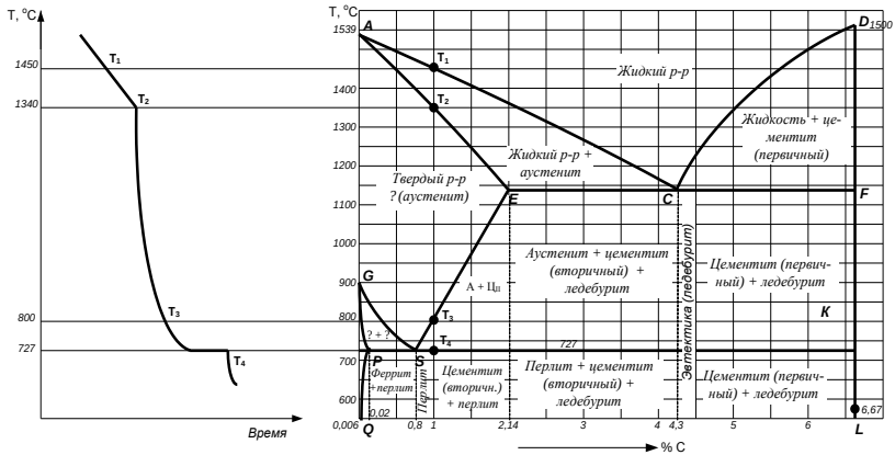
Рис.1.6.Диаграмма состояния Fe-Fe 3 C и кривая кристаллизации, соответствующая содержанию углерода в стали 1 %
