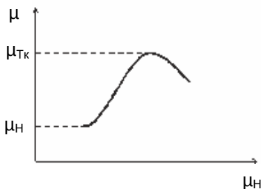
Рис. 1.6. Зависимость относительной магнитной проницаемости ферромагнетиков от напряженности магнитного поля
