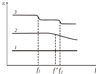
Рис. 1.8. Частотная зависимость \varepsilon диэлектриков с мгновенной (1) и релаксационными (2, 3) видами поляризации
