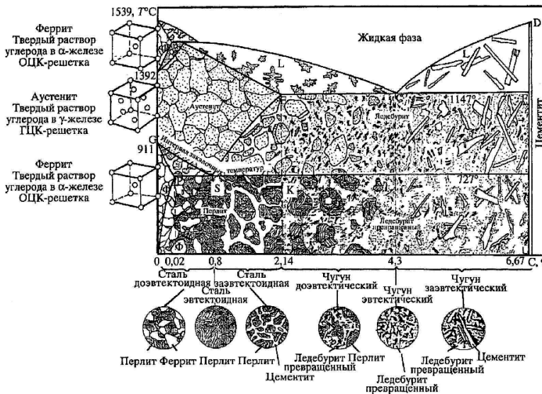
Рис. 1.7. Диаграмма состояния сплава железо - цементит
