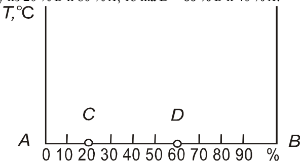
Рис. 1.16. Координаты для изображения диаграммы состояния двухкомпонентной системы
