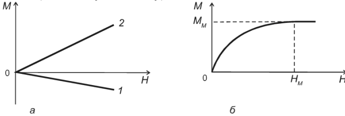
Рис. 2.2. Зависимость намагниченности M от напряженности магнитного поля H : а – для диамагнетиков (1) и парамагнетиков (2); б – для парамагнетиков при низких температурах или очень сильных полях
