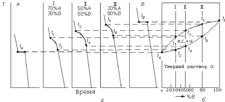
Рис. 1.3. Построение диаграммы состояния сплавов для случая неограниченной растворимости компонентов A и B в твердом состоянии: а – кривые охлаждения; б – диаграмма состояния
