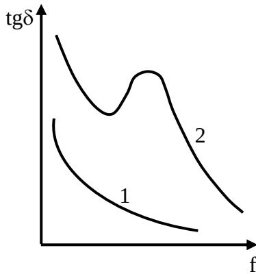
Рис. 4. Частотная зависимость \operatorname{tg} \delta для диэлектриков с потерями на сквозную электропроводность (1); с потерями на электропроводность и поляризационными потерями (2)
