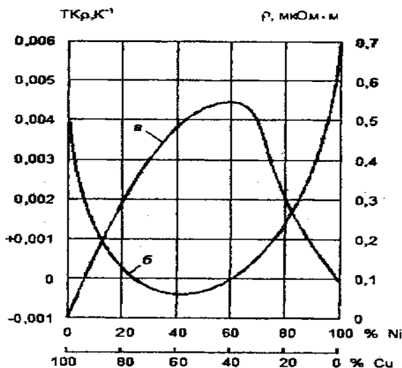
Рис. 4. Зависимость \rho (а) и ТКР (б) сплавов системы Cu-Ni от состава (в процентах по массе) [1]
