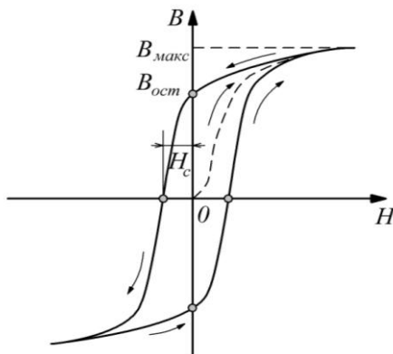
Рис. 3. Зависимость индукции от напряженности магнитного поля ферромагнетиков (петля гистерезиса), ( H_c – коэрцитивная сила; B_{\text{ост}} – остаточная индукция)
