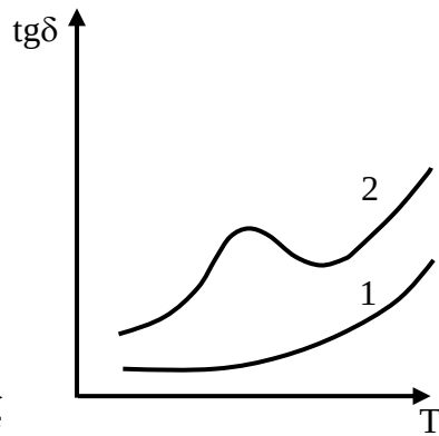
Рис. 5. Зависимость \operatorname{tg} \delta от температуры для непольярных (1) и полярных (2) диэлектриков
