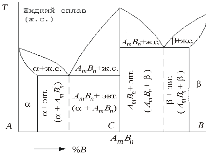
Рис. 1.5. Диаграмма состояния сплавов для случая образования компонентами A и B сплава - химического соединения
