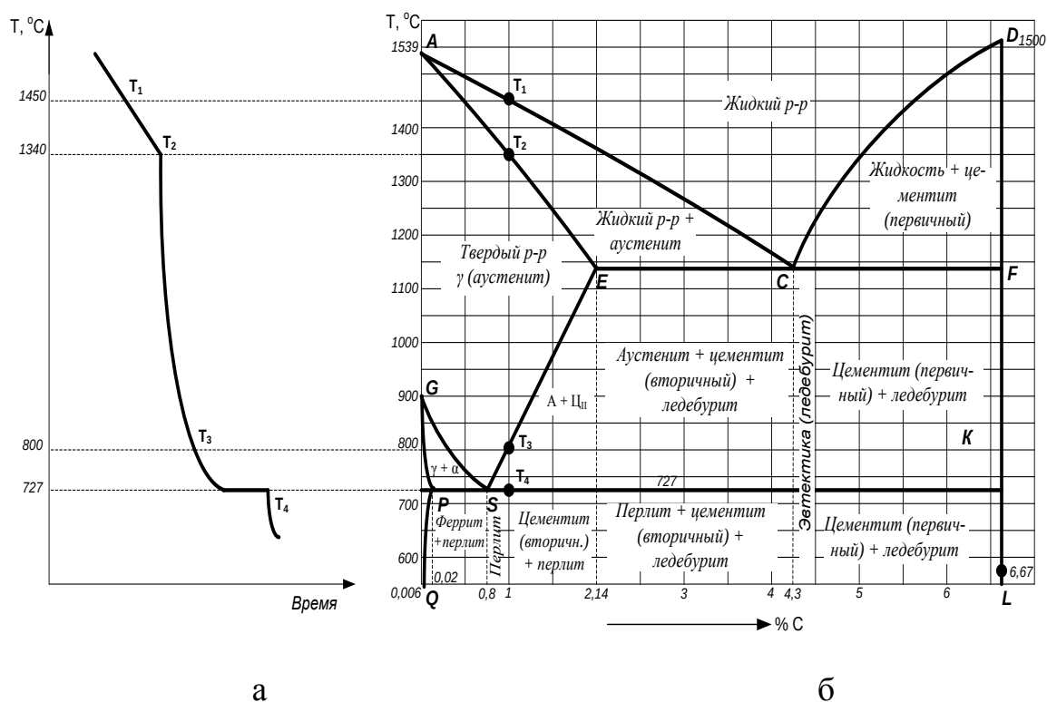
Рис.1.2. Кривая охлаждения (а) и иллюстрация на диаграмме состояния изменений фазового состояния стали, содержащей 1% углерода, происходящих при медленном охлаждении от 1600 до 20 ^{\circ}\text{C} (б)
