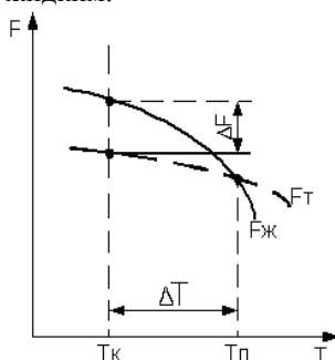
Рис. 1.9. Изменение энергии Гельмгольца F (свободной энергии) металла в жидком F_{ж} и твердом F_{т} состояниях в зависимости от температуры ( T_k — температура, при которой происходит кристаллизация)
