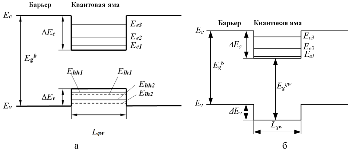
Рис. 2. Энергетическая диаграмма КРС с КЯ и зонной диаграммой I типа (а) и II типа (б)
