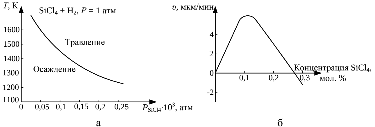
Рис. 4.1. Граница областей роста и травления кремния в системе \text{SiCl}_4\text{--H}_2 в зависимости от температуры и парциального давления P_{\text{SiCl}_4} (а) и зависимость скорости роста эпитаксиального слоя \text{SiCl}_2 ( T = 1170^\circ\text{C} ) (б)
