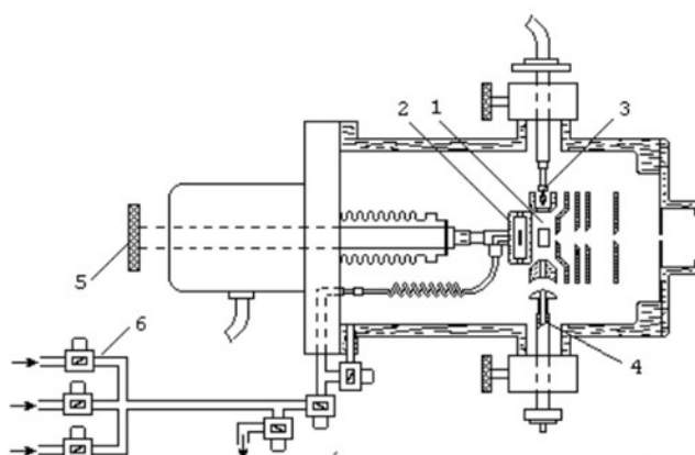
Схема комбинированного источника ЭИ и ХИ
