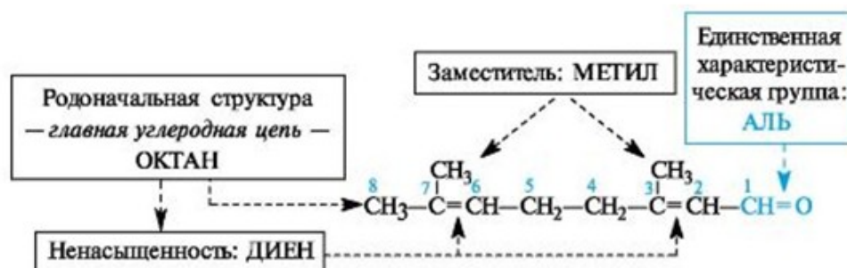
3,7-диметилоктадиен-2,6-аль
