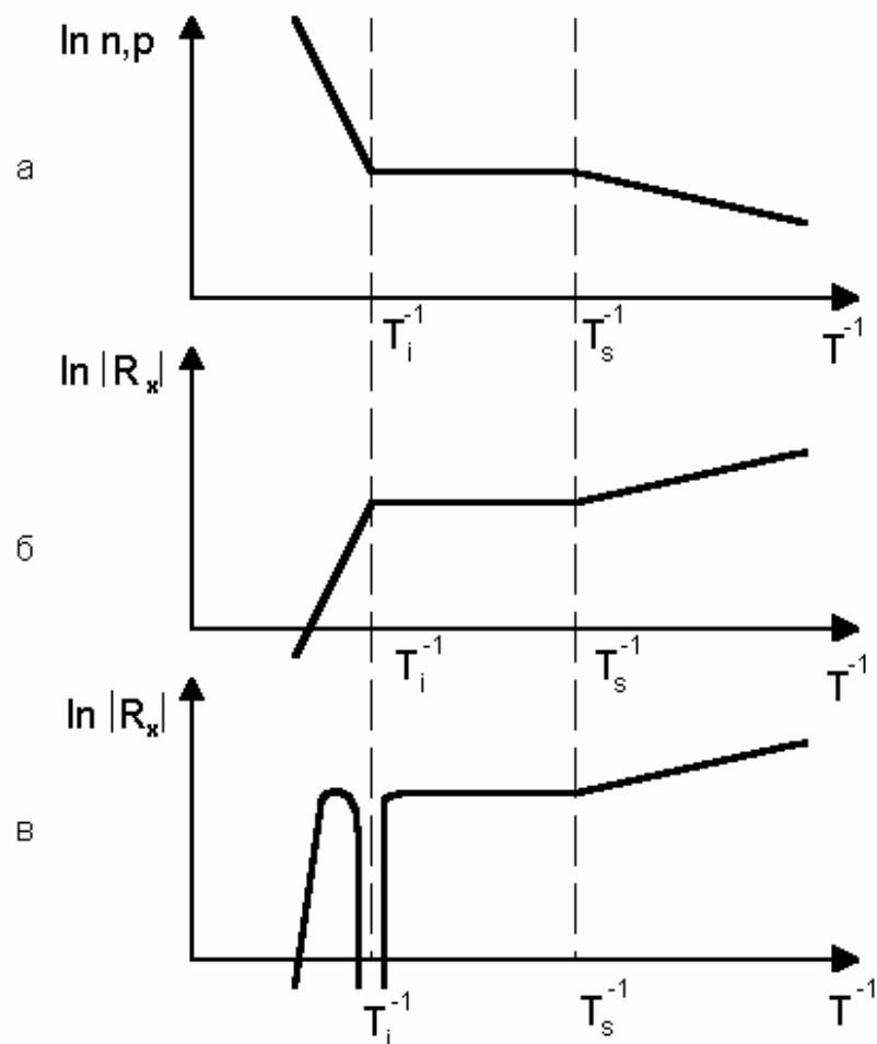
Рис. 2.19. Зависимость концентрации носителей заряда (а) и коэффициента Холла для полупроводника n-типа (б) и полупроводника p-типа (в)
