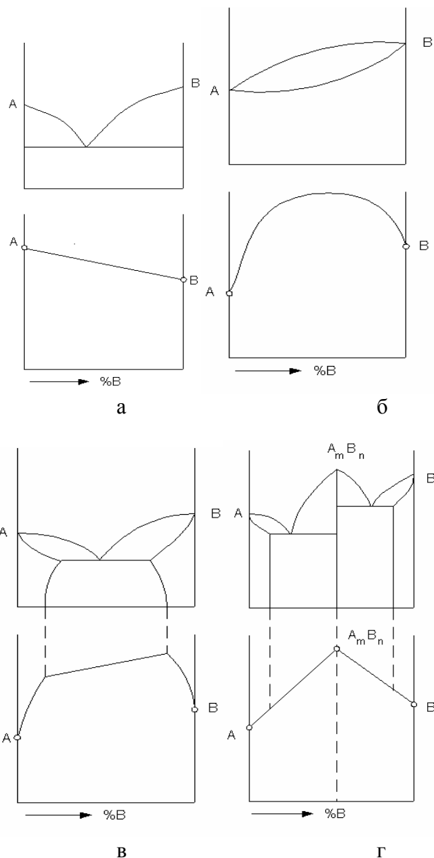
Рис. 1.10. Свойства сплавов и вид их диаграммы состояния (по Н.С. Курнакову)
