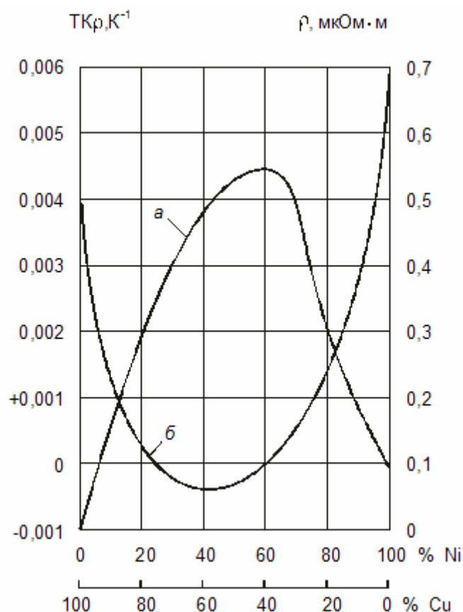
Рис. 1.15. Зависимость \rho (а) и ТК \rho (б) сплавов системы Cu-Ni от состава (в процентах по массе)
