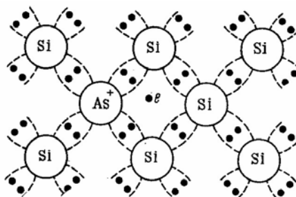
Рис. 2.5. Плоская модель кристаллической решетки полупроводника n-типа (кремния, легированного мышьяком)
