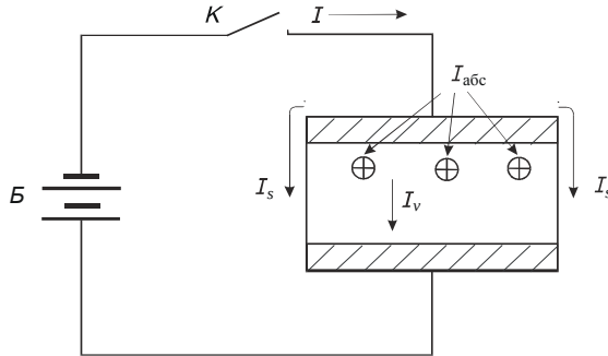
Рис. 1.1. Виды электрического тока в образце диэлектрика: I – общий ток изоляции; I_{абс} – ток абсорбции; I_v – объемный ток; I_s – поверхностный ток
