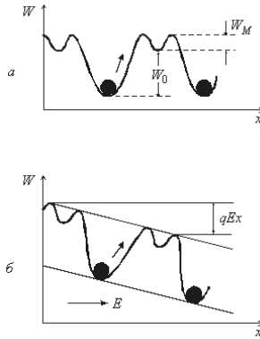
Рис. 1.3. Модель ионной проводимости твердых диэлектриков: а – без внешнего поля; б – понижение потенциального барьера W_0 на величину qEx при наложении электрического поля напряженностью E ( W_M – глубина междуузельной потенциальной ямы)
