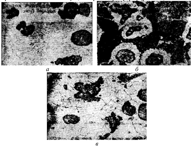
Рис. 2.7. Микроструктура высокопрочного чугуна с шаровидным графитом, х 250: а – нетравленный шлиф; б – феррито-перлитный чугун; в – ферритный чугун
