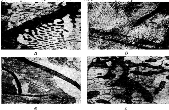
Рис. 2.5. Микроструктура серого чугуна: а – чугун со структурой ледебурит – перлит – графит; б – перлитный чугун; в – феррито-перлитный чугун; z – ферритный чугун
