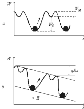
Рис. 1.3. Модель ионной проводимости твердых диэлектриков: a – без внешнего поля; б – понижение потенциального барьера W_0 на величину qEx при наложении электрического поля напряженностью E ( W_M – глубина междуузельной потенциальной ямы)
