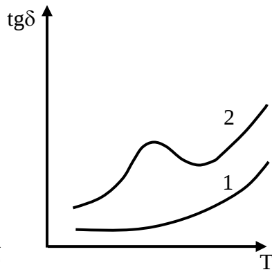
Рис. 5. Зависимость \operatorname{tg} \delta от температуры для неполярных (1) и полярных (2) диэлектриков
