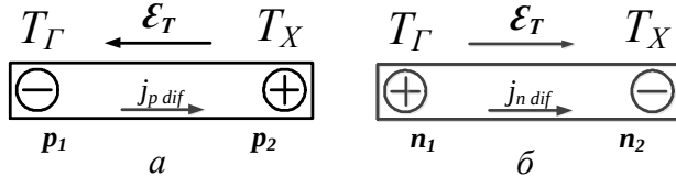
Рис. 1. Возникновение термо-ЭДС в полупроводниках: a – полупроводник n-типа; b – полупроводник p-типа ( T_T > T_X , p_1 > p_2 , n_1 > n_2 )
