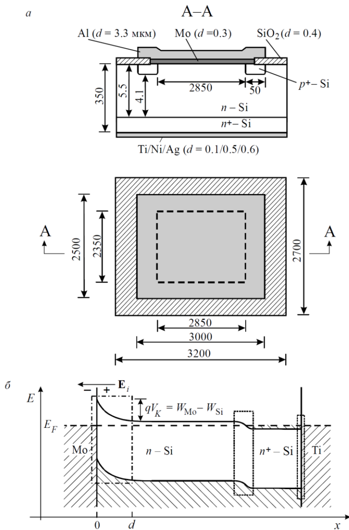
Рис. 4. Диод Шоттки: a – виды в плане и разрезе (размеры даны в мкм, S \approx 6.7 \text{ мм}^2 ); б – энергетическая зонная диаграмма
