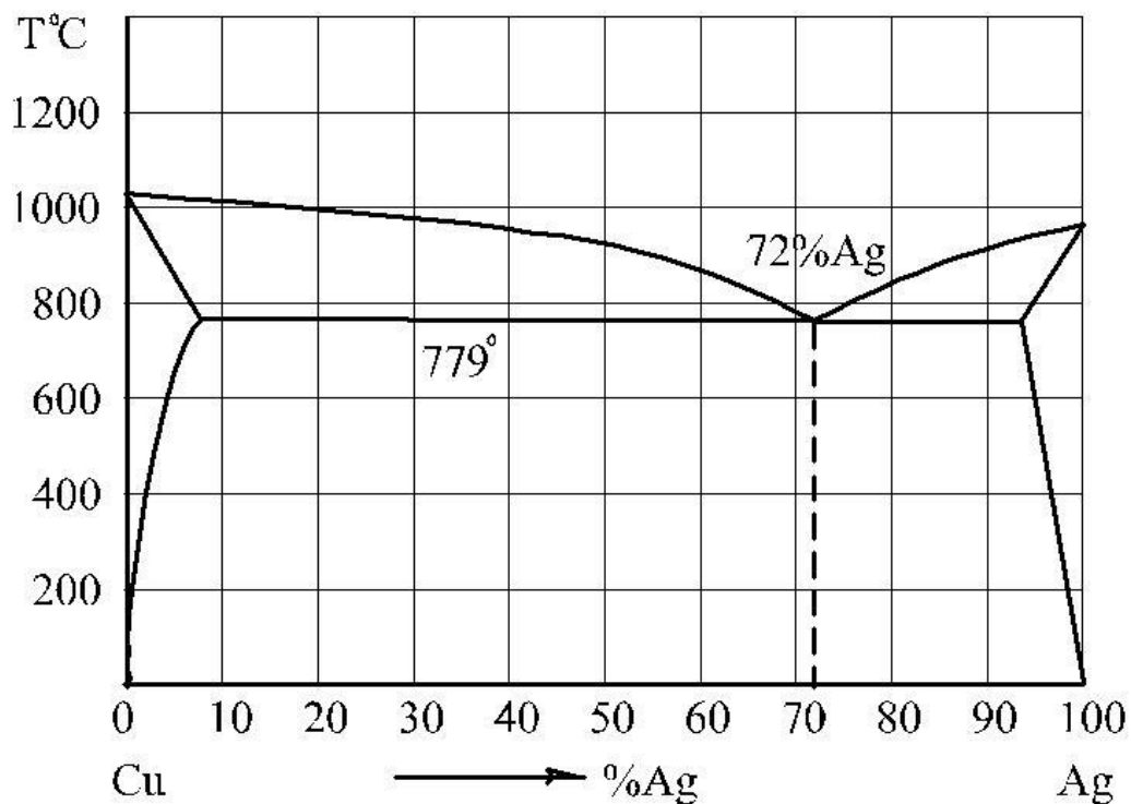
Рис. П1. Диаграмма состояния системы «медь – серебро»
