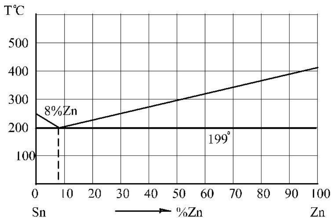
Рис. П6. Диаграмма состояния системы «олово – цинк»
