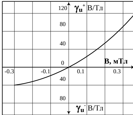
Рис. 6. Зависимость вольтовой магнитной чувствительности полярного магнитотранзистора от индукции магнитного поля при I_b = 0,2 \text{ мА} и I_{К-Э} = 120 \text{ мкА}
