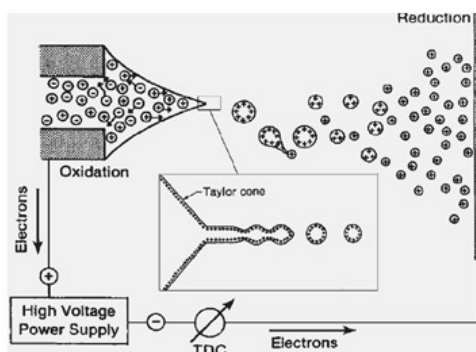
Принцип электрораспыления
