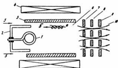
Схема газоразрядного источника ионов
