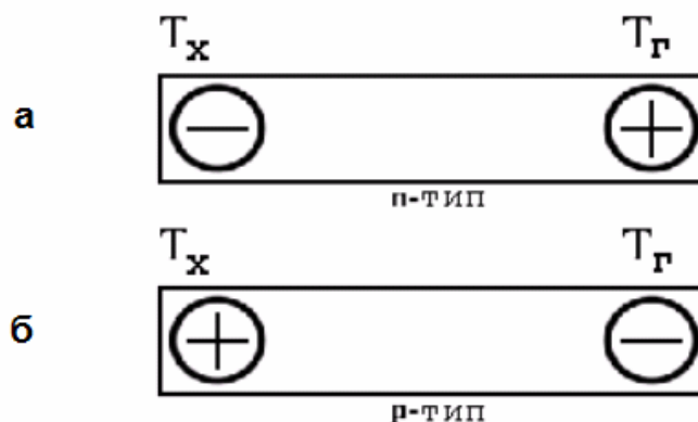
Рис. 2.15. Объемные заряды в полупроводнике n-типа (а) и р-типа (б) при наличии разности температур
