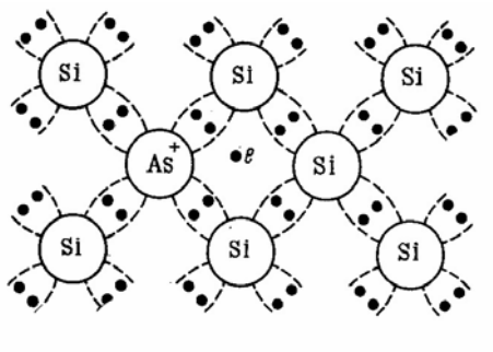
Рис. 2.5. Плоская модель кристаллической решетки полупроводника n-типа (кремния, легированного мышьяком)
