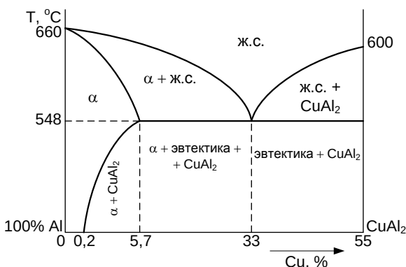
Рис. 3.1. Диаграмма состояния сплава Al–Cu
