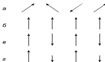
Рис. 1. Схематическое расположение спинов в парамагнитных ( a ), ферромагнитных ( б ), антиферромагнитных ( в ) и ферримагнитных ( г ) веществах. Диамагнетикам свойственна полная взаимная компенсация магнитных моментов атомов.
