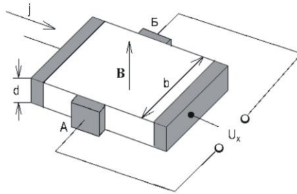
Рис. 6. Образец для измерения э.д.с. Холла
