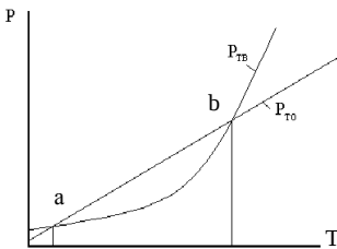
Рис. 1. Зависимости мощности выделения тепла ( P_{\text{ТВ}} ) и мощности отвода тепла ( P_{\text{ТО}} ) от температуры
