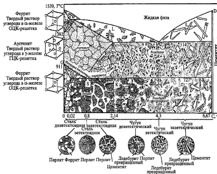
Рис. 1.7 Основные фазы на диаграмме состояния железо - углерод
