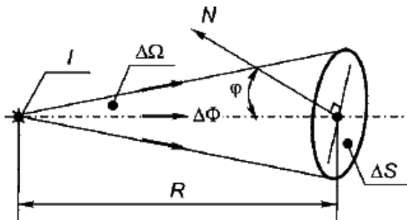
Рис. 2. Определение освещенности [1]
