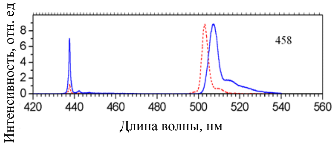
ZnCdS/ZnSSe, КЯ второго типа (Расчет для спектра, обозначенного сплошной линией)
