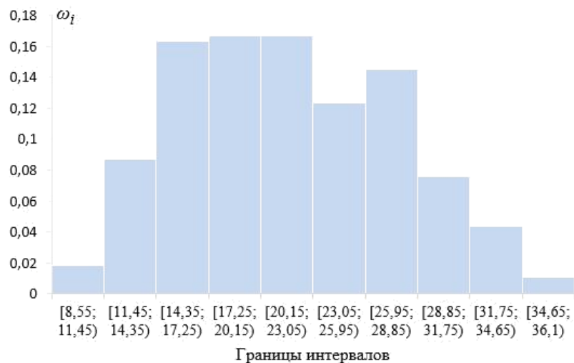
Рисунок 2 – Гистограмма частот
