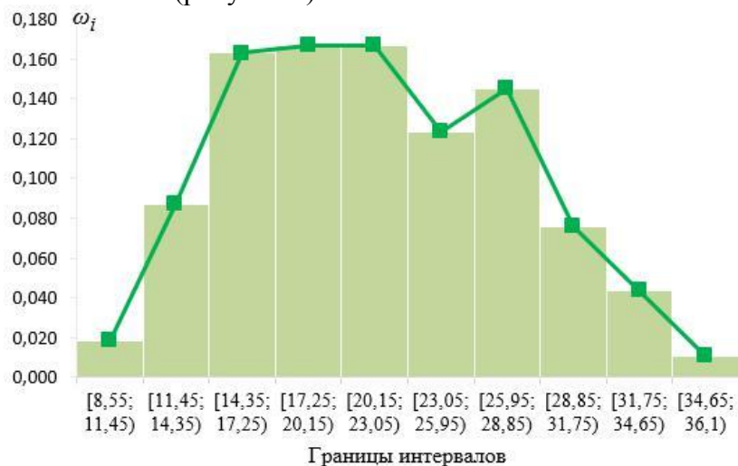
Рисунок 3 – Гистограмма и полигон частостей
