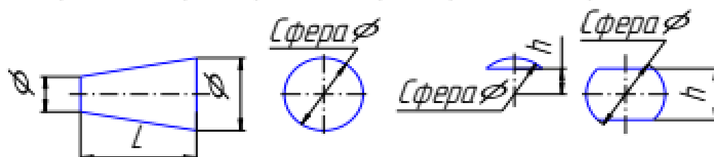
Усечённый конус Шар Шаровой сегмент Шаровой слой
