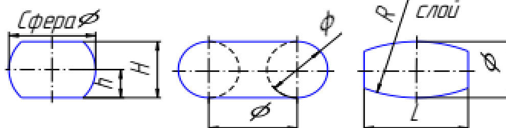
Шаровой слой Тор (кольцо) Тор (бочка)
