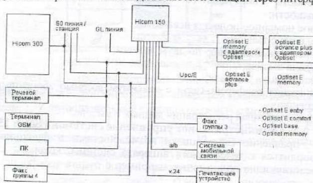
Рис. 2.2. Интерфейсы и абонентские устройства станции Нисом 150Е
