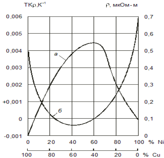
Рис. 1.2. Зависимость \rho (а) и \text{TK}\rho (б) сплавов системы Cu-Ni от состава (в процентах по массе)
