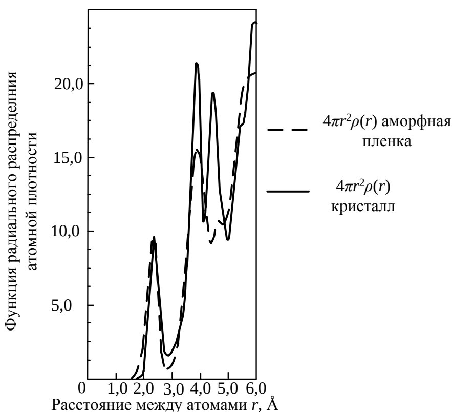
Рис. 4. Радиальная функция распределения электронной плотности, полученная с помощью дифракции электронов на тонкой кремниевой аморфной пленке (пунктирная линия) и той же пленке после рекристаллизации (сплошная линия) [27]
