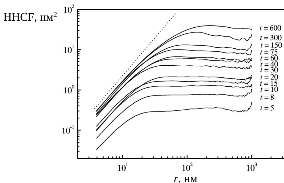
Рис. 10. Парные корреляционные функции в зависимости от времени осаждения пленок a-Si:H. Время осаждения указано в минутах [54]
