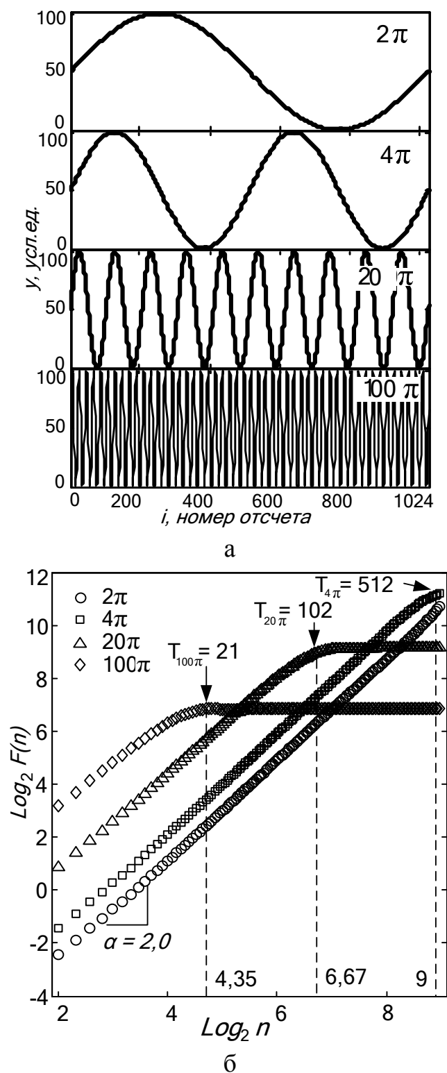
Рис. 16. Иллюстрация эффекта кроссовера флуктуационной функции по методу DFA на примере реализаций синусоидальной формы: а – реализации синусоиды с различным числом периодов; б – зависимость флуктуационной функции от масштаба [стрелками показаны точки кроссовера, которые соответствуют значениям масштаба разбиения, равным длине колебаний T (в шкале отсчетов) каждой реализации. Слева от кроссовера значение скейлингового показателя \alpha равно 2, справа \alpha = 0 ]
