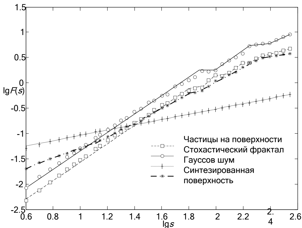
Рис. 24. Исследование средней флуктуационной функции в зависимости от масштаба для модельной поверхности, построенной по принципу сходства с поверхностью неупорядоченного полупроводника
