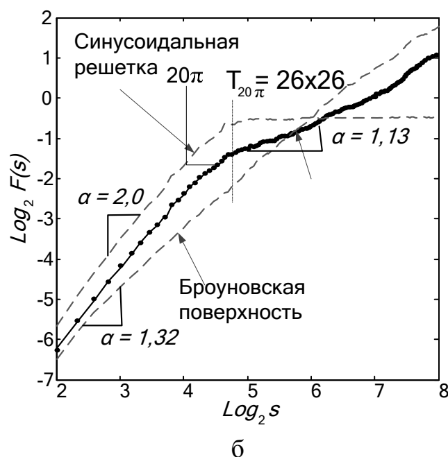
Рис. 22. Пример формирования кроссовера при сложении двух поверхностей с различными скейлинговыми показателями: а – исходные поверхности: синусоидальная решетка с кроссовером на T=26 \times 26 пикселей и броуновская поверхность с \alpha=1,3 ; б – флуктуационные функции всех процессов. Видно, что итоговый процесс (синтезированная поверхность) является промежуточным вариантом между периодической и шумовой составляющей: одновременно обладает и кроссовером с \alpha=2 и выраженным самоподобием во всем диапазоне масштабов, унаследованных от броуновской поверхности
