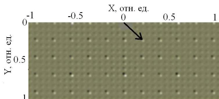
Рис. 11. Распределение СВИ для поверхности фрактала «Ковер Серпинского»
