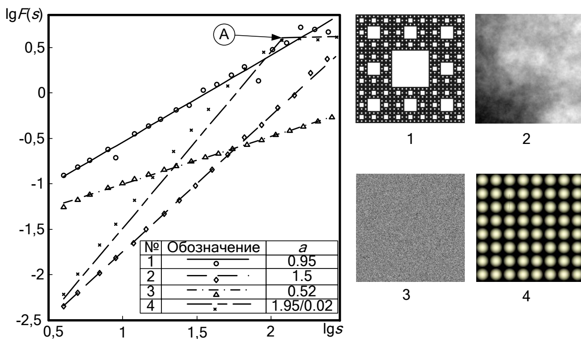
Рис. 18. Расчет скейлингового показателя для модельных поверхностей: 1 – «Ковер Серпинского», 2 – броуновская поверхность, 3 – гауссов шум; 4 – «Кластеры»
