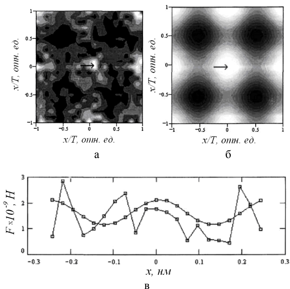
Рис. 8. Изображение условной решетки атомов углерода, полученное численным моделированием, и результат ее вейвлет-фильтрации: а – искаженное шумом изображение модельной решетки атомов углерода; б – изображение, полученное после построчной вейвлет-фильтрации; в – силовые сигналы вдоль отдельных линий сканирования [52]
