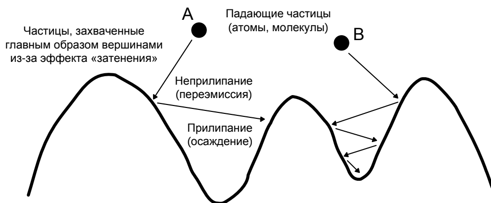
Рис. 3. Поверхность растущей тонкой пленки при эффектах затенения и переэмиссии [19]
