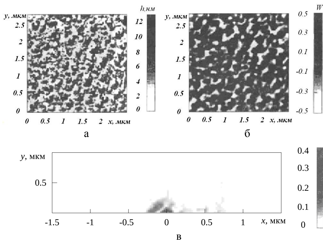
Рис. 9. Структурная диагностика поверхности с помощью корреляционного и вейвлет-анализа: а – исходное изображение рельефа поверхности; б – ее вейвлет-преобразование с характерными параметрами структур, полученными из анализа АКФ; в – АКФ [53]
