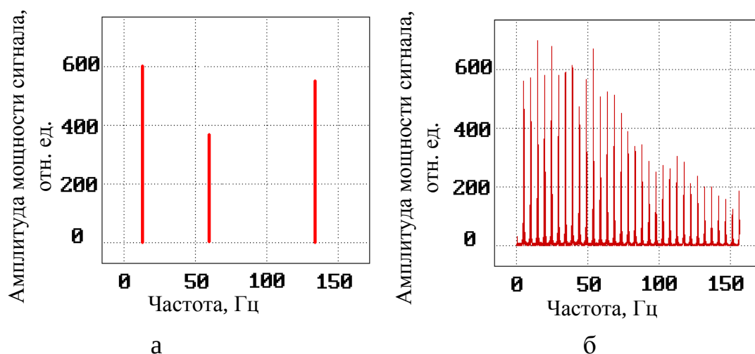
Рис. 7. Типичный Фурье-спектр: для линейной системы (а); для поверхности неупорядоченного материала (б) [49]
