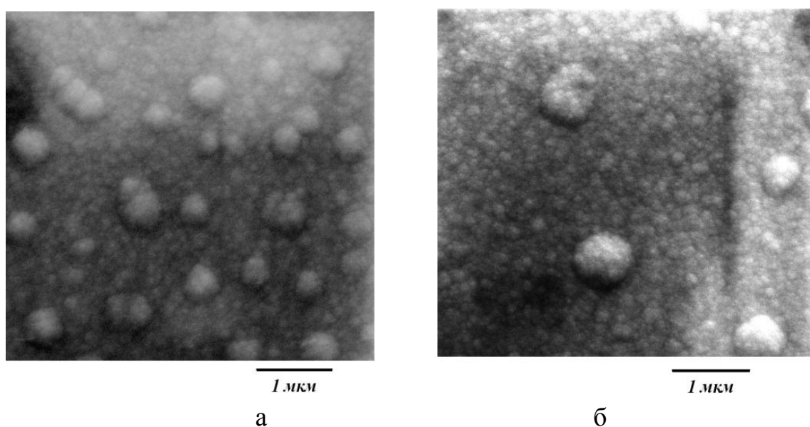
Рис. 5. РЭМ-изображения поверхности образцов a-Si:H, полученных методом ТР: а – при температуре подложки 220°C и времени осаждения 5 часов; б – при температуре подложки 170°C и времени осаждения 5 часов [45]
