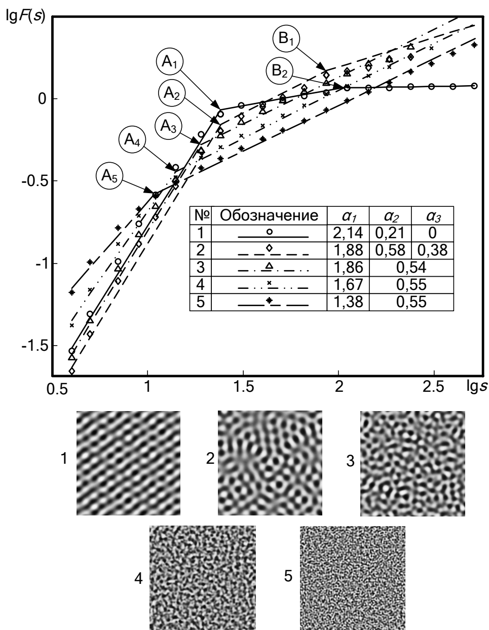
Рис. 20. Исследование средней флуктуационной функции в зависимости от масштаба для спектрально синтезированных поверхностей с вариацией длины автокорреляции
