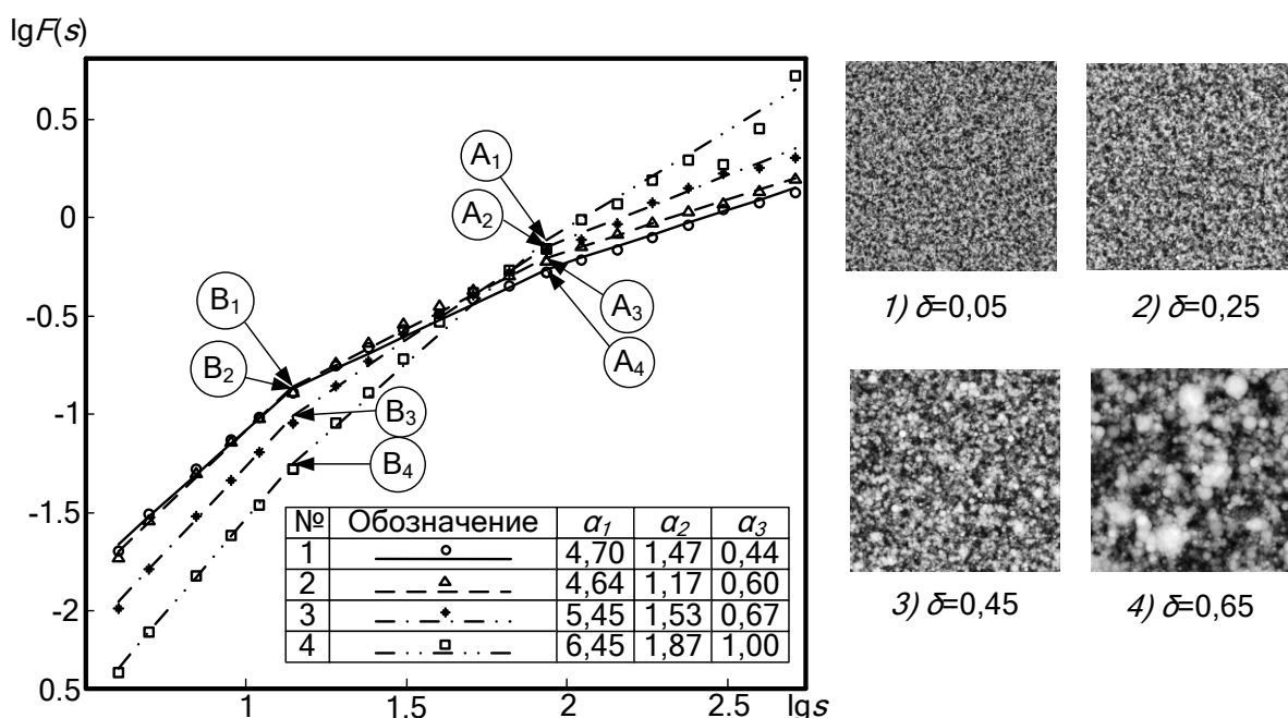
Рис. 19. Исследование флуктуационной функции в зависимости от масштаба для модельной поверхности «Частицы» с вариацией разброса среднего размера трехмерных образований на поверхности
