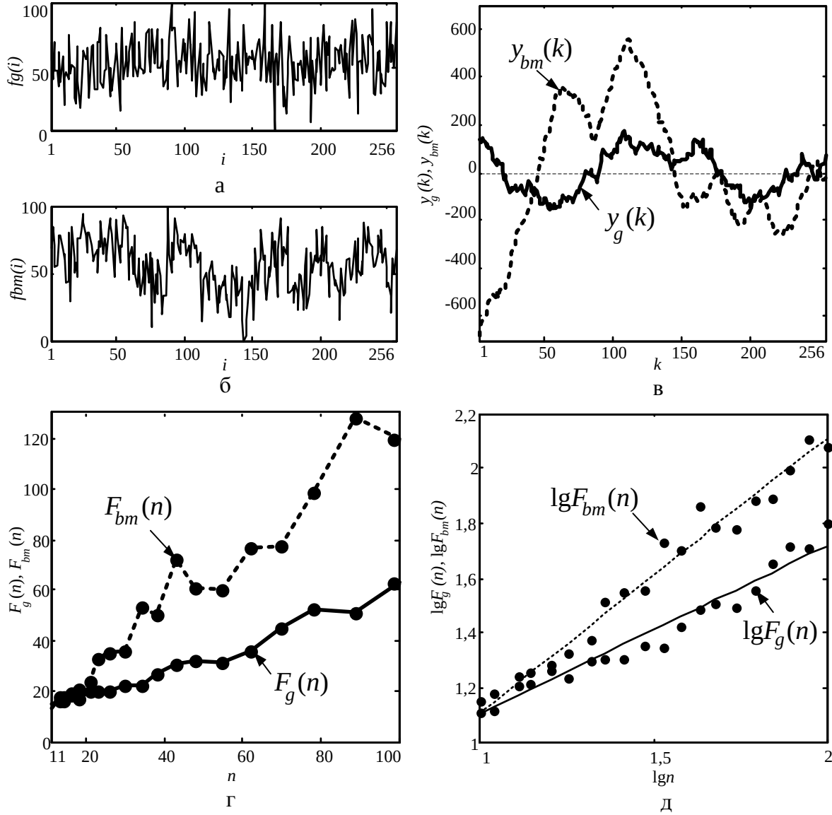
Рис. 13. Иллюстрация работы алгоритма DFA на моделях гауссова шума и одномерного броуновского движения: а – профиль гауссова шума; б – профиль броуновского шума; в – суммированный сигнал гауссова y_g(k) и броуновского шума y_{bm}(k) ; г – среднеквадратическая ошибка линейной аппроксимации гауссова F_g(n) и броуновского шума F_{bm}(n) ; д – логарифмическое представление флуктуационной функции
