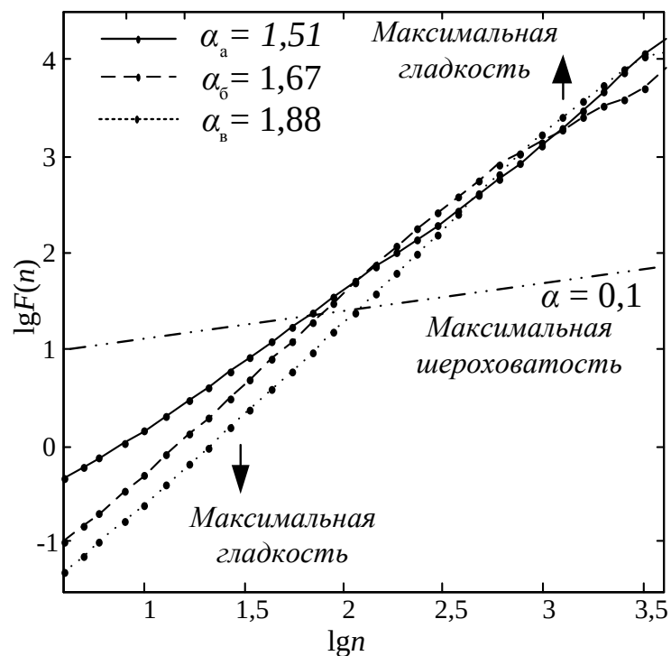
Рис. 15. Демонстрация повышения значения \alpha для более “гладких” реализаций по сравнению с “изрезанными”: а – реализации случайного фрактала типа броуновского движения с различными степенями сглаживания скользящим окном; б – расчет скейлингового показателя \alpha для данных реализаций
