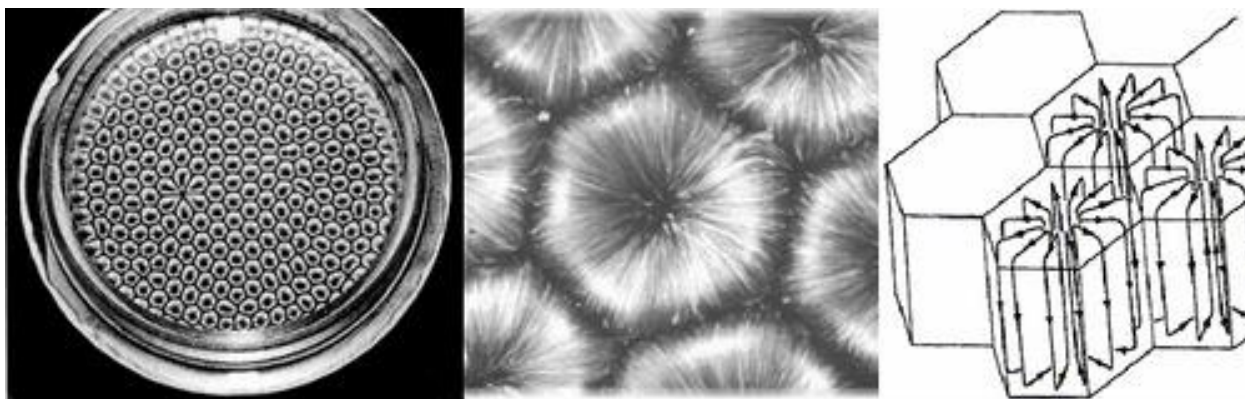
Рис. 2. Ячейки Бенара: а – снимок в реальном масштабе, б – снимок в увеличенном масштабе, в – схема потоков жидкости в отдельных ячейках [13]
