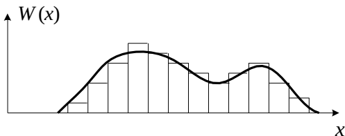
Рисунок 4 –Сглаженная гистограмма
